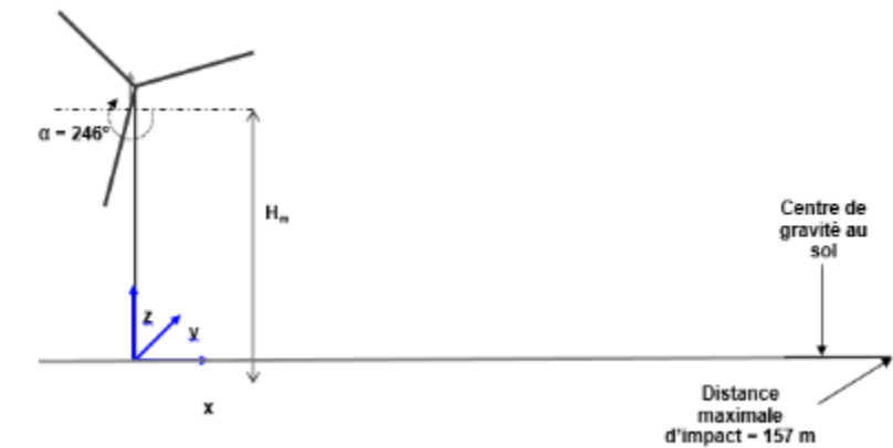
Figure 73 : Illustration de la parabole du centre de gravité de la pale dans le cas n°1 (configuration 1)
