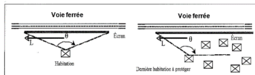
Figure 83 : Dimensionnement des protections acoustiques
