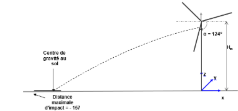
Figure 73 : Illustration de la parabole du centre de gravité de la pale dans le cas n°1 (configuration 1)
