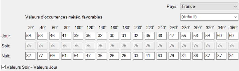
Figure 80 : Valeurs d'occurrences météorologiques maximales favorables entre les villes de Montpellier et Perpignan
