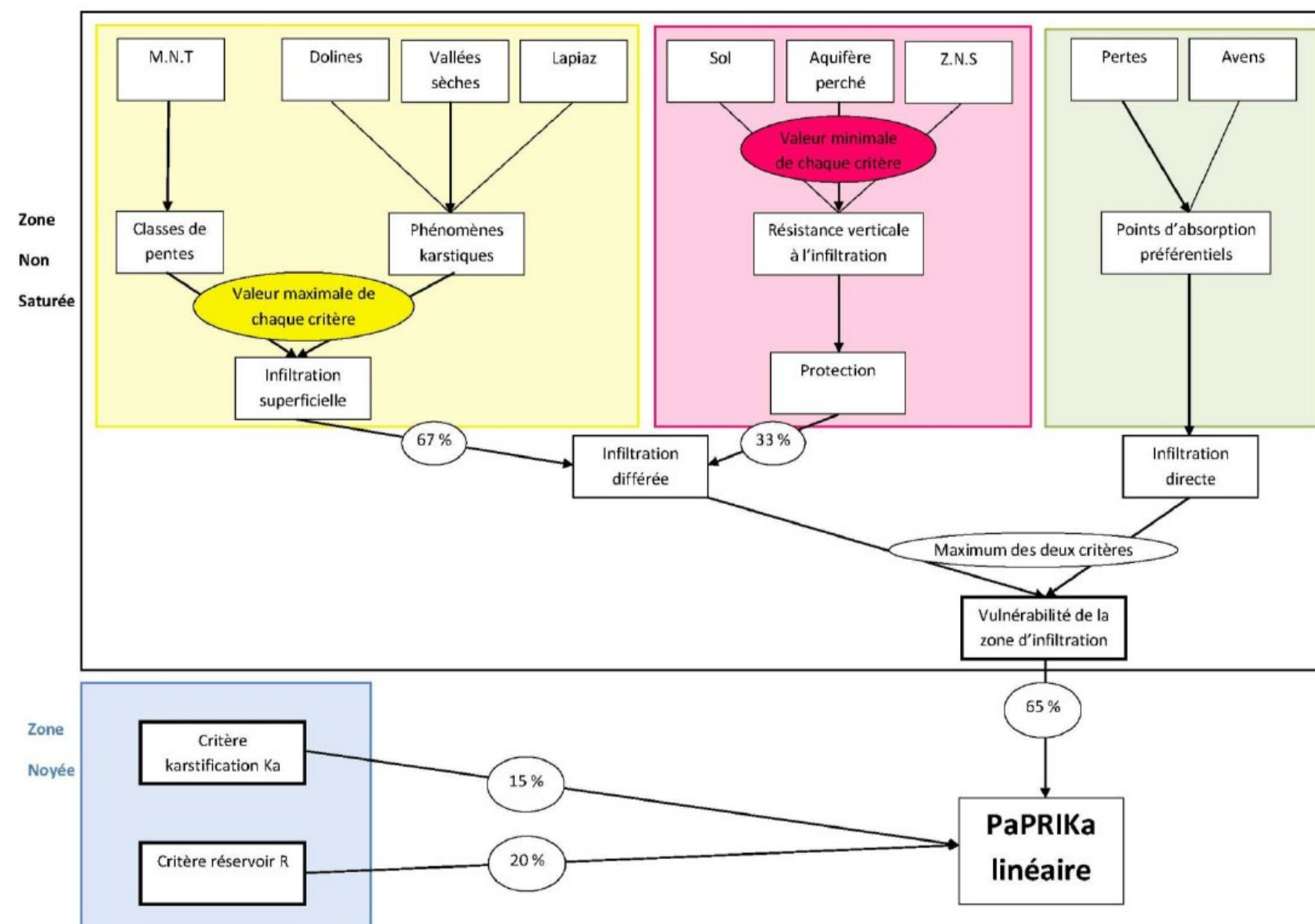
Figure 35 : Schéma de l'adaptation de la méthode PaPRIKa
