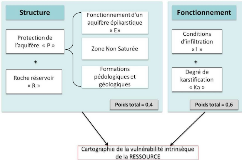
Figure 31 : Conceptualisation du karst dans la méthode PaPRIKa
