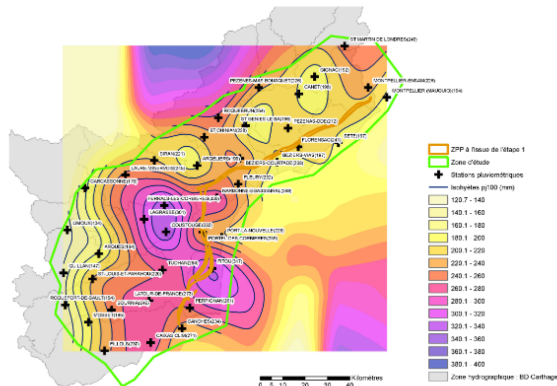
Figure 42 : Isohyètes de la pluie journalière centennale (1999 inclus)
